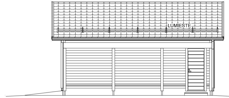
JULKISIVU KAAKKOON
