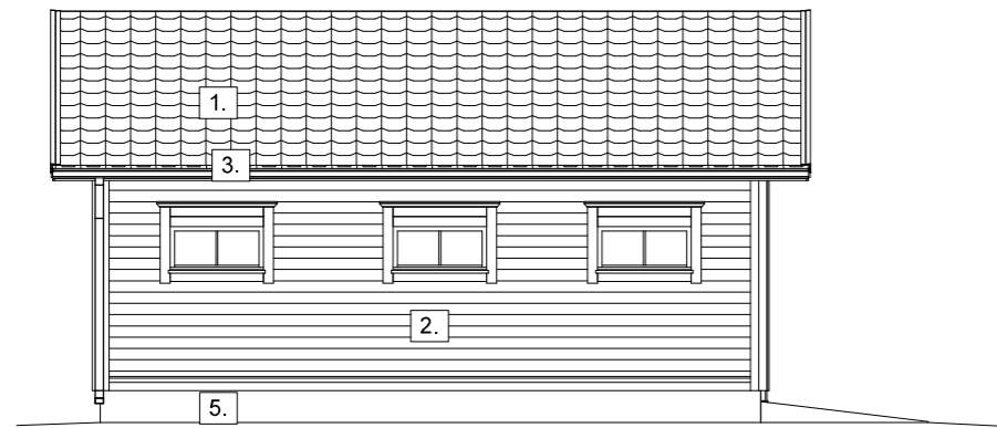
JULKISIVU LUOTEeseen
