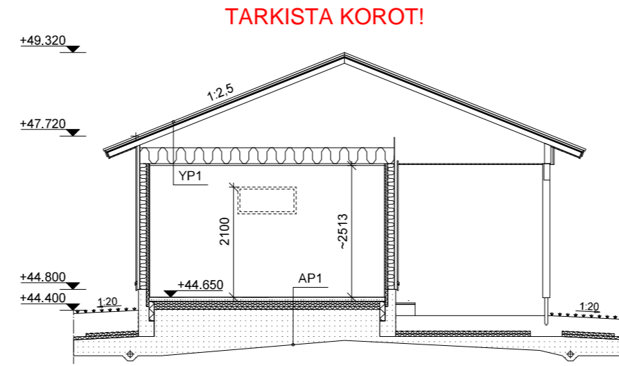
LEIKKAUS A-A
